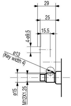
Kurbelwellentyp
