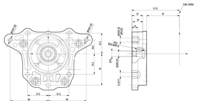
Flansch
